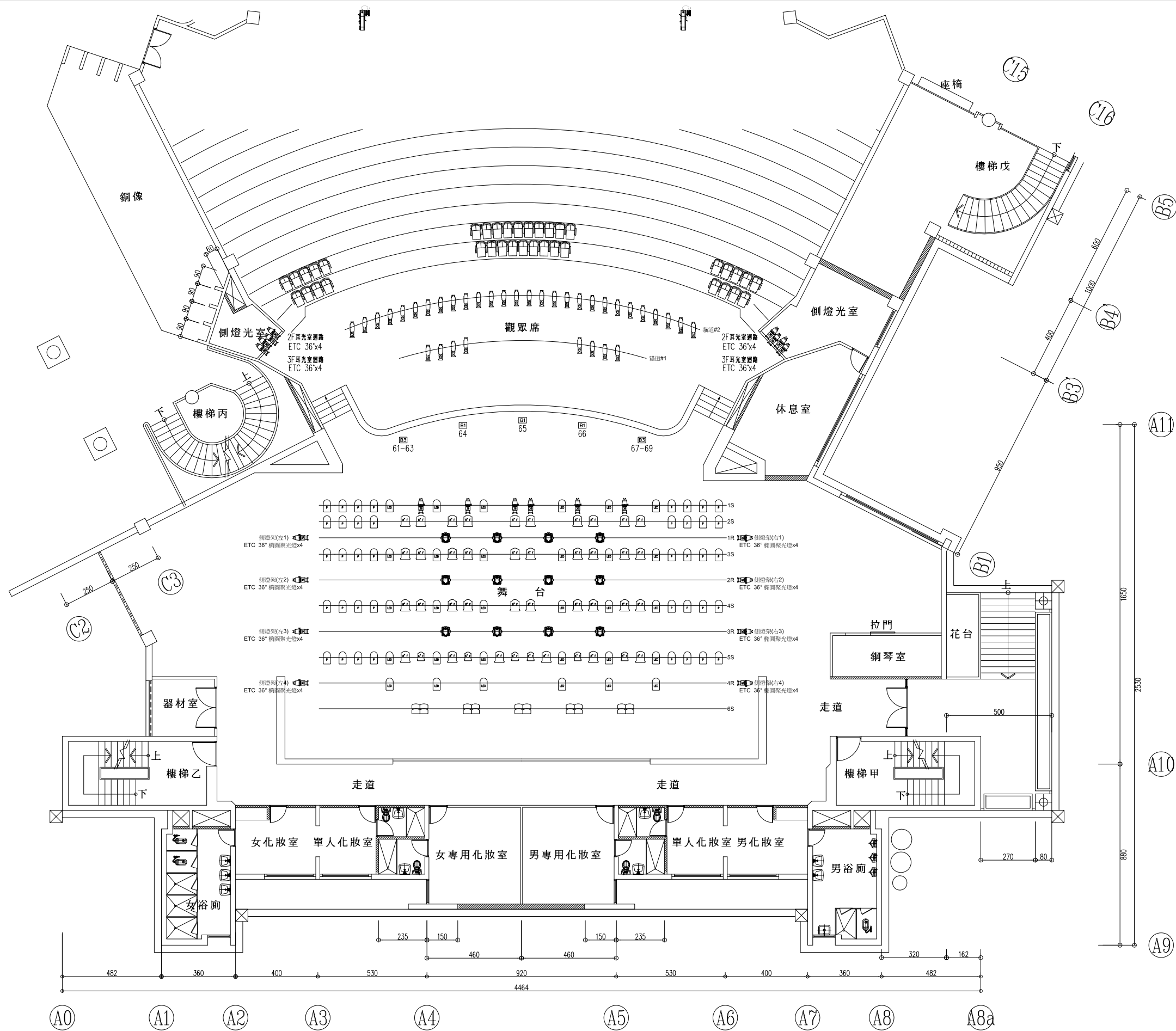
舞台燈光燈具配置平面圖
